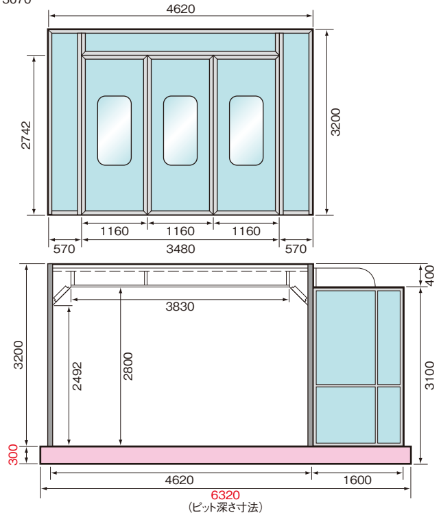
正面寸法
