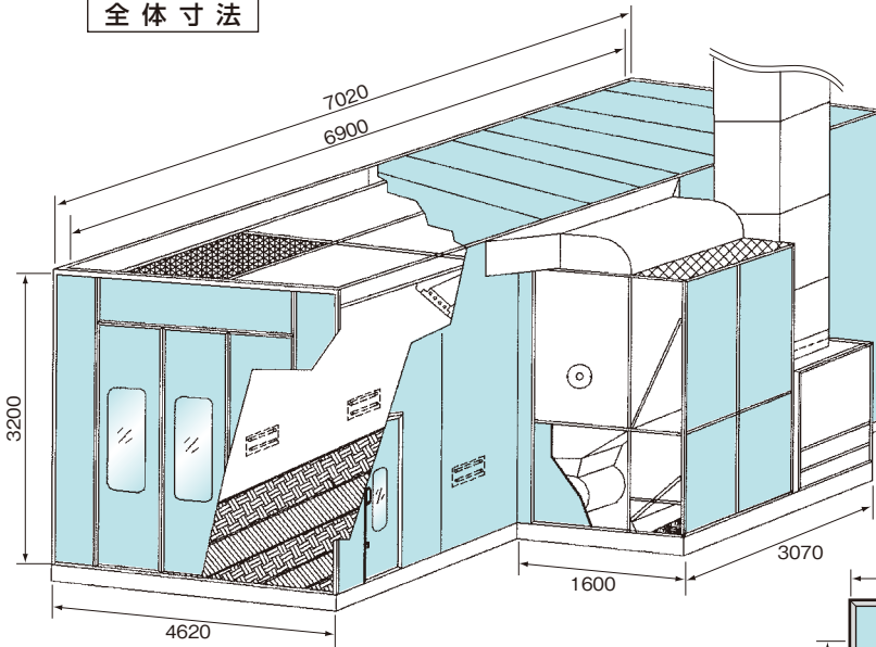
全体寸法
