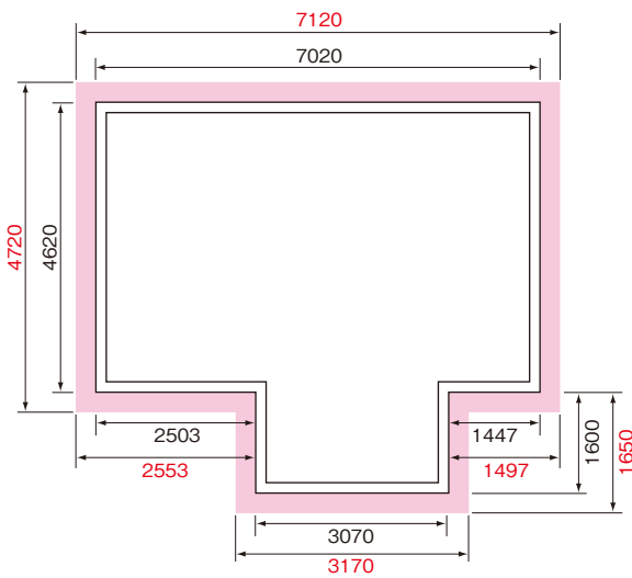
ピット寸法
